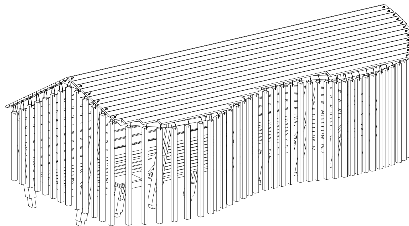
6 Installation des suspentes verticales de 60x60mm
