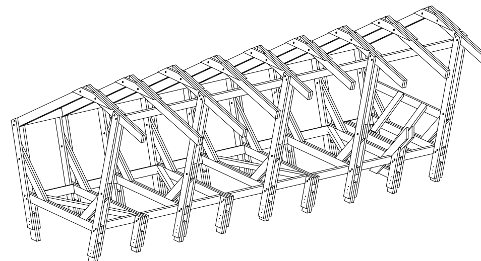
3 Assemblage de l'ensemble des portiques
