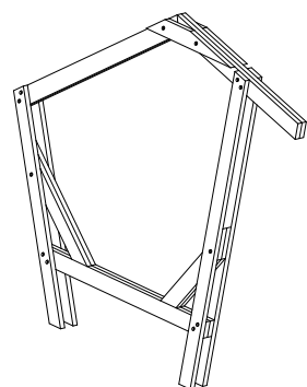
1 Fabrication des portiques moisés chevillés en atelier en planches de 100x27mm
