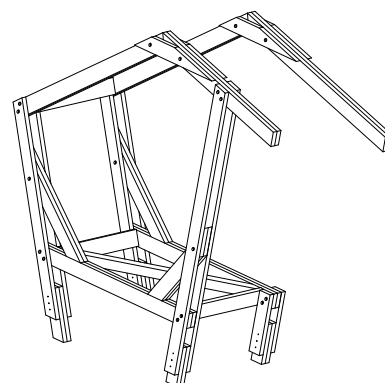
2 Assemblage de 2 portiques et réglage des pieds
